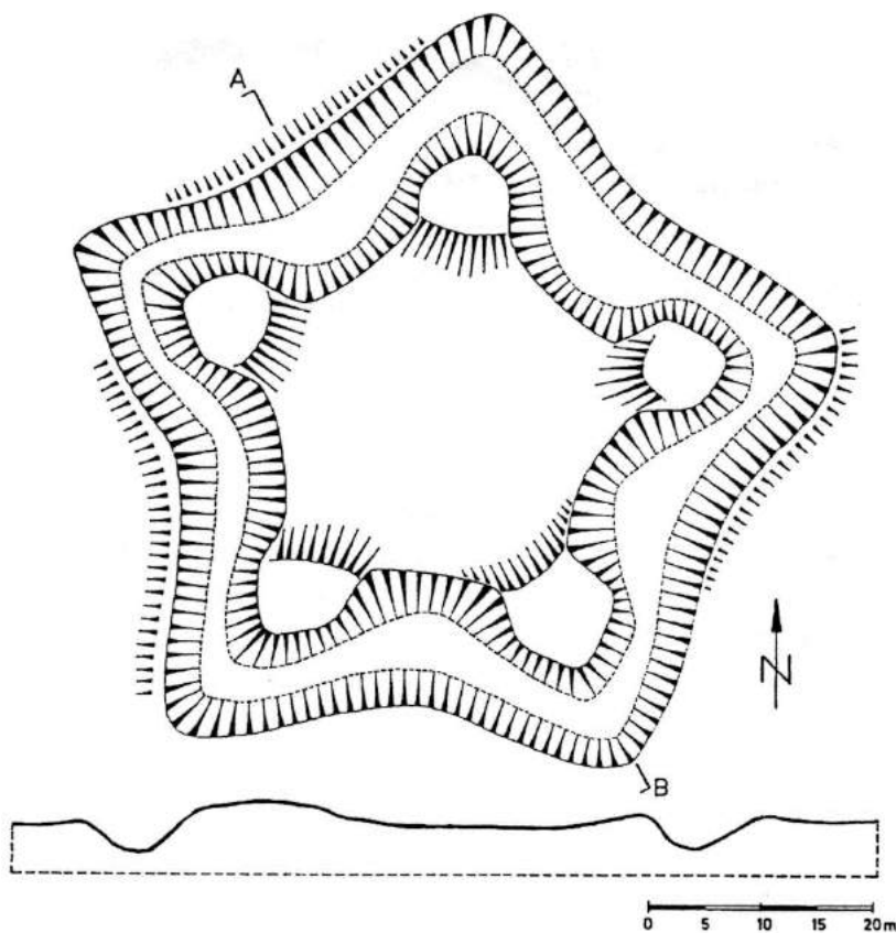
Abbildung 3 Grundrissplan der sternförmigen Schanze (nach Timpel/Grimm 1975, Abb. 24)
